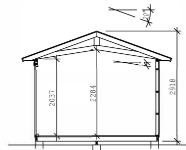
SEKTION
